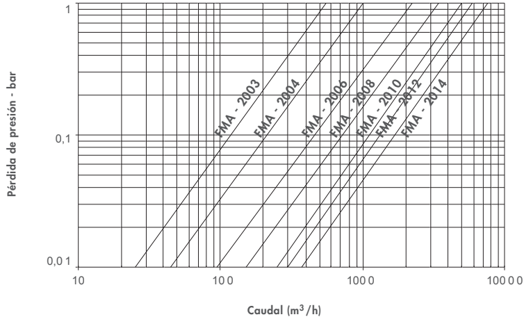
Pérdida de carga FMA-2000-INOX-1500 MICRAS
